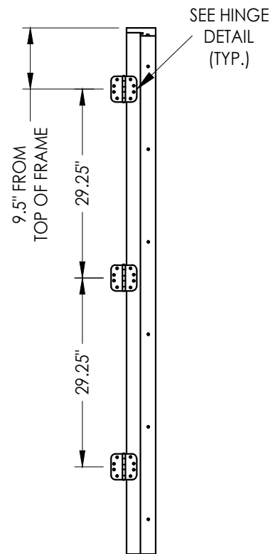
HINGE JAMB
